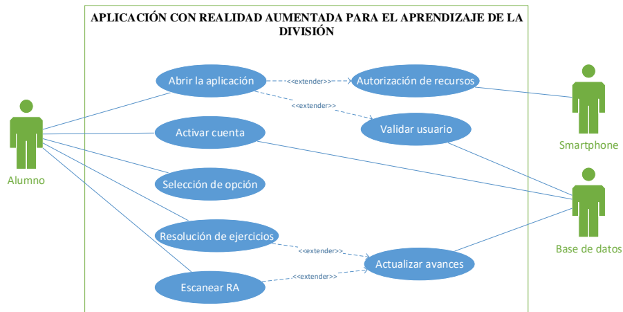
Figura 1. Caso de uso. Fuente (elaboración propia).
