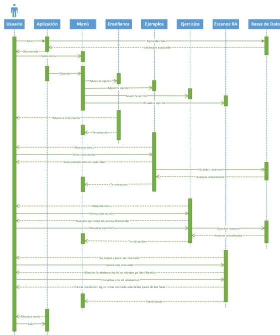
Figura 3. Diagrama de secuencia. Fuente (elaboración propia).
