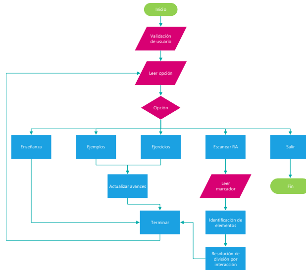
Figura 2. Diagrama de funcionamiento. Fuente (elaboración propia).
